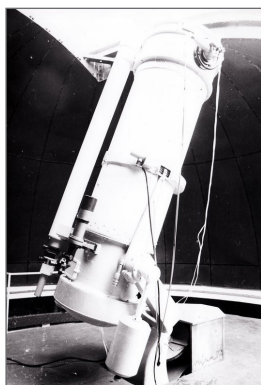
Obr. 2.2: Dalekohled observatoře Masarykovy univerzity o průměru 60 cm s fotonásobičem v Newtonově ohnisku
