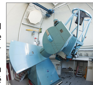
Obrázek 1.3: Dalekohled DK-154 na observatoři La Silla v Chile.
