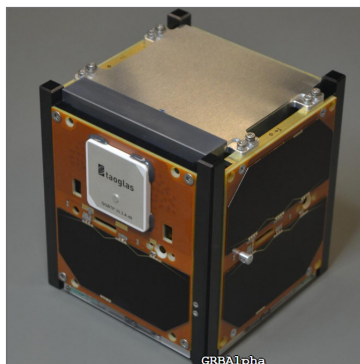
Obr. 2.10: Nanosatelit GRBAlpha pro detekci záblesků gama
