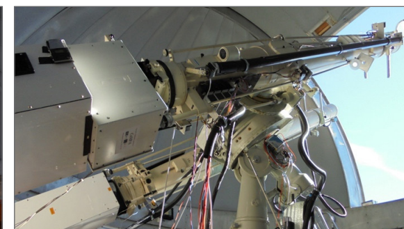
Obr. 5.6: Koronograf s COMP-S (od r. 2011) v popredí a s CCD v pozadí
