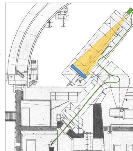
Obrázek 1.1: Schéma dalekohledu spolu s naznačenou cestou světla optickým vláknem k přístrojům.
