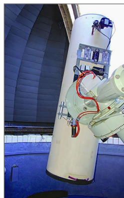
Obr. 5.11: 61-cm Newton / od r. 2000
